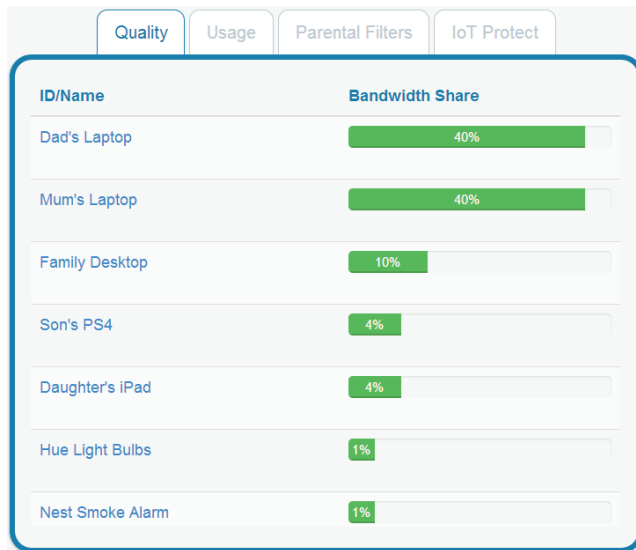
Fig. 9. QoE control.
